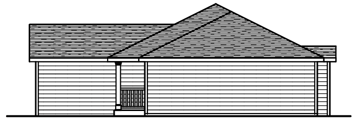
RIGHT ELEVATION
